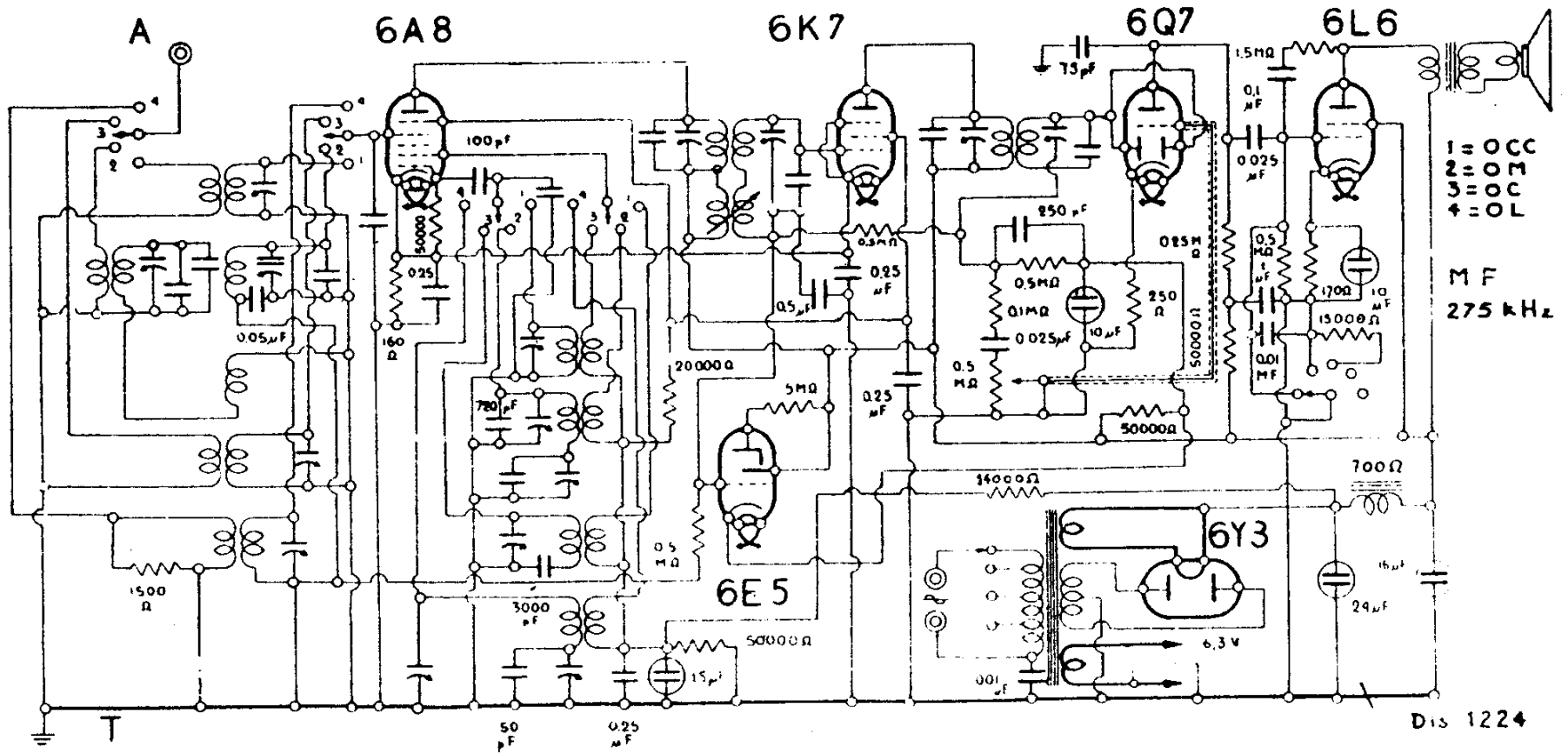
IRRADIO - MOD. « D X 7 »
